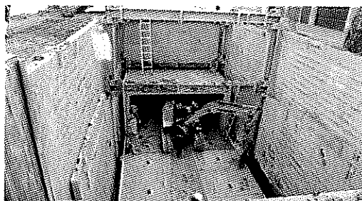
Posa del Nuovo Collettore di Levante III st.
