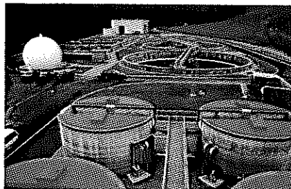
Vista di insieme dell'impianto di depurazione di Monguelfo
